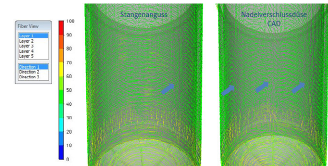
Spritzgießsimulation Strukturanalyse (Glasfaserorientierungen)
