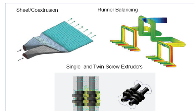
Strömungsanalyse
