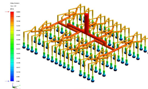
Auslegung eines Heißkanals für ein 96-fach-Werkzeug
