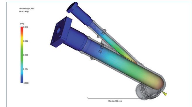
Spritzgießsimulation von Kernversatz
