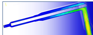
Simulation einer Nadelverschlussdüse im Profil
